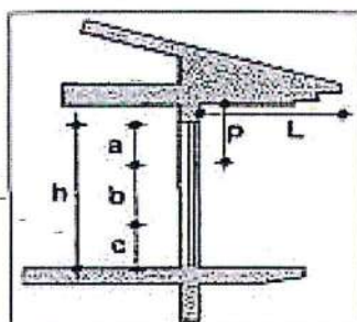
Figura 1 - SCHEMA ESPLICATIVO DELLA SUPERFICIE ILLUMINANTE UTILE.
